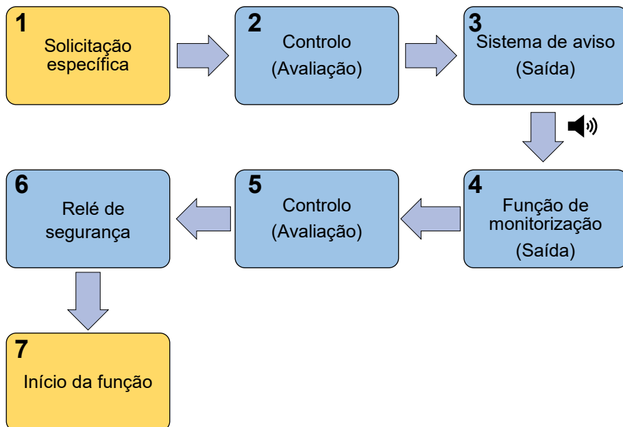
Fig. 5 Sistema de aviso acústico quando a função de segurança é solicitada num momento específico
