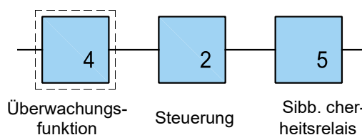
Abb. 8 Sicherheitsrelevantes Blockdiagramm
