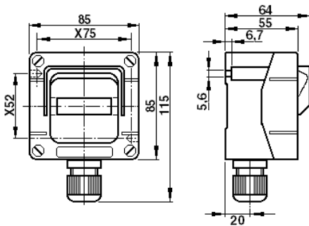
Maßbild Maße in mm
