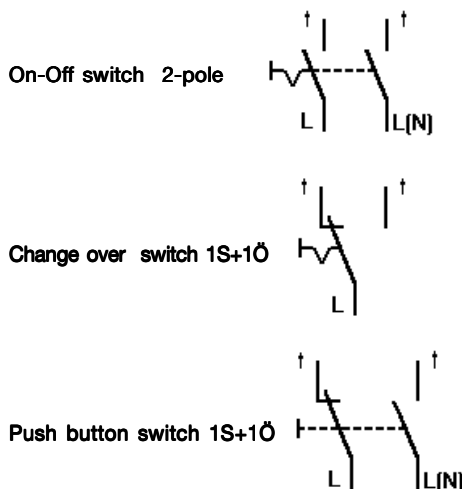
Wiring diagrams
